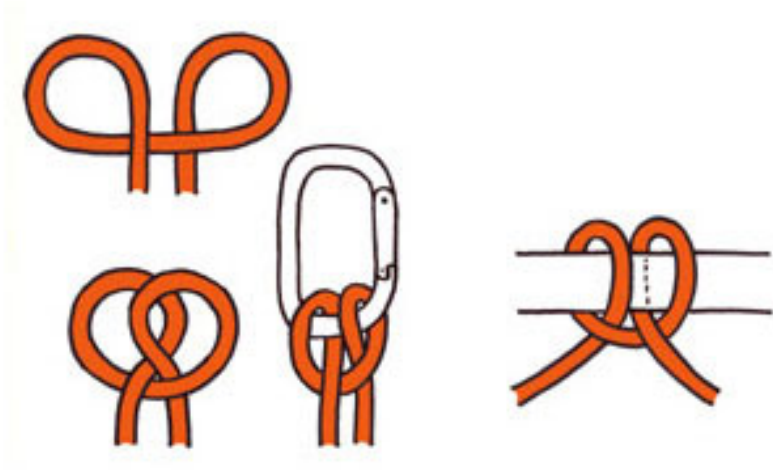
Lodní smyčka
